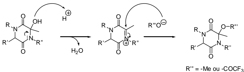
Schéma 154 : Piégeage de l'acyliminium par le solvant
