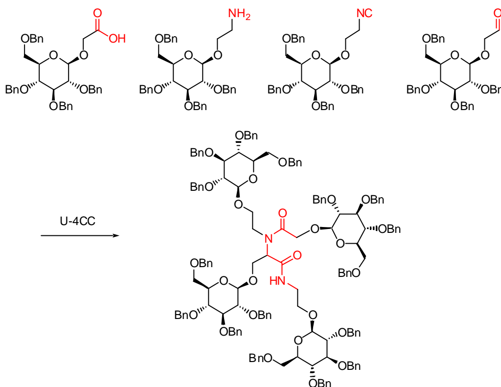
Schéma 29 : Synthèse de molécules tétraglycomimétiques
