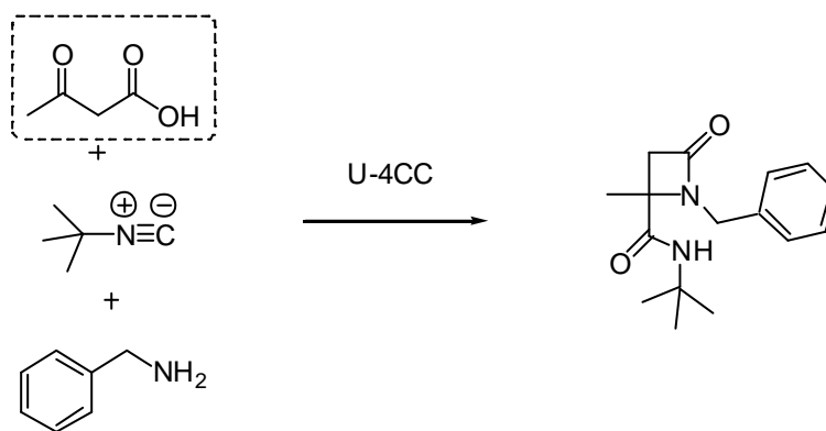
Schéma 146 : Utilisation d'un \beta -cétoacide dans la condensation de Ugi
