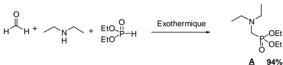
Schéma 121 : Formation d' \alpha -aminophosphonates
