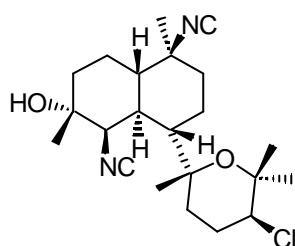
Kalihinol A
