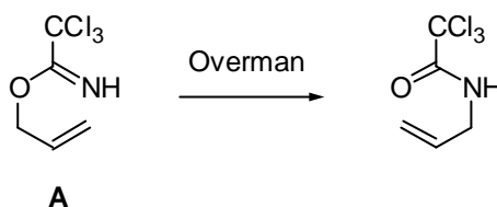
Schéma 41 : Réarrangement de type Overman
