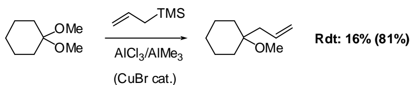
Schéma 131 : Alkylation d'acétals
