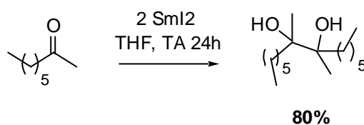
Schéma 102 : Pinacolisation de cétones avec le diiodure de samarium
