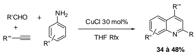
Schéma 91 : Formation de quinoléines
